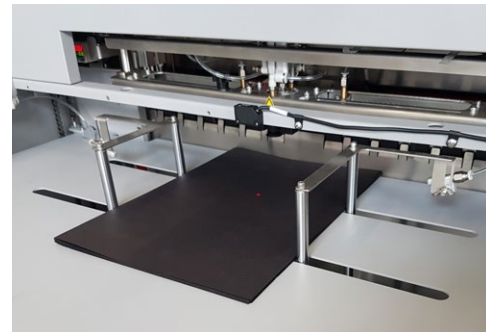
Integrierter Zwischenpappenanleger
